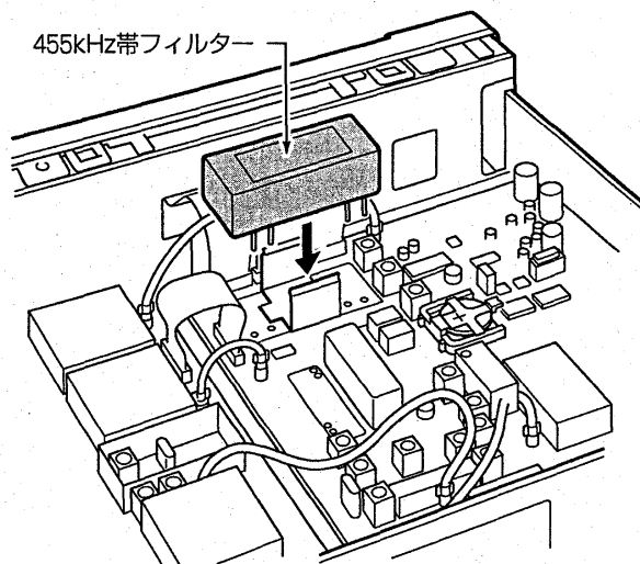
●455kHz帯フィルターの取り付けかた
