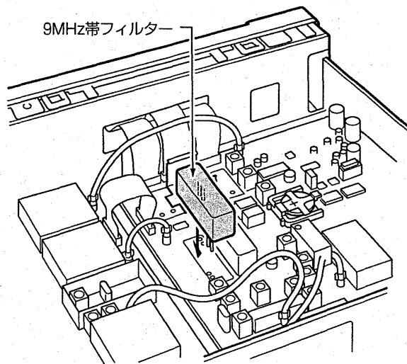
●9MHz帯フィルターの取り付けかた
